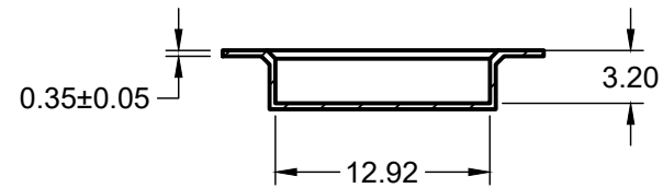
SECTION A-A SCALE 2:1
