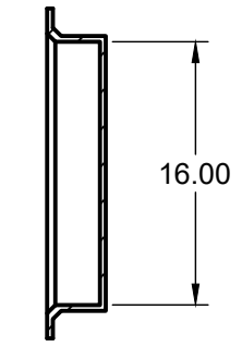
SECTION B-B SCALE 2:1
