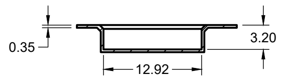
SECTION A-A SCALE 2:1
